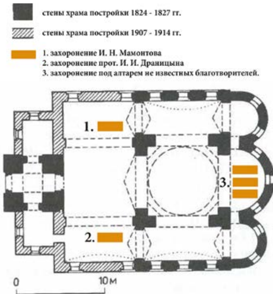
План храма Похвалы Пресвятой Богородицы в Ратмино после расширения 1907 - 1914 гг.
